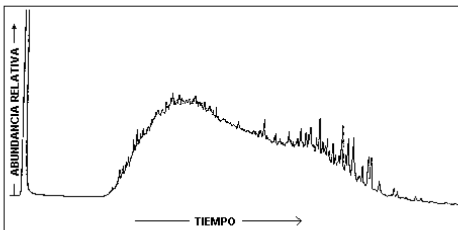
Cromatograma de la fracción saturada del mene de Mene de Mauroa (Tomado de: Del Olio, 1993)
