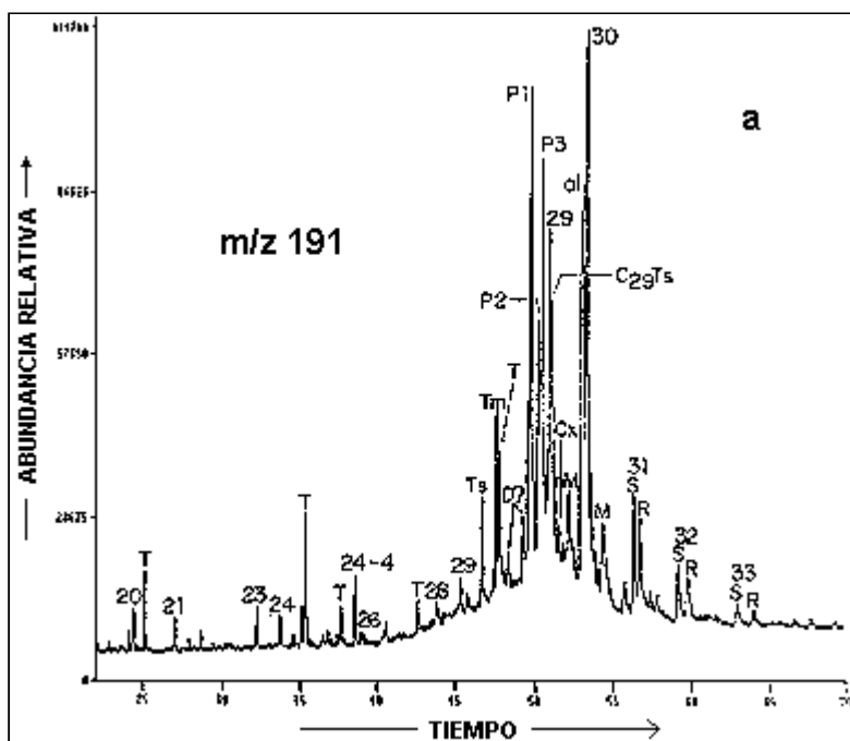
Cromatograma de la fracción saturada del mene de Mene de Mauroa (Tomado de: Del Olio, 1993)
