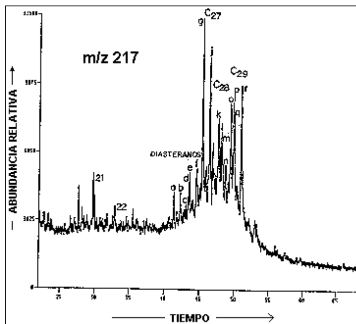
Distribución de biomarcadores esteranos m/z 217 del mene Mene de Mauroa (Tomado de: Del Olio, 1993)
