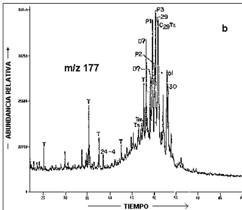
Distribución de biomarcadores terpanos m/z 191(a) y m/z 177(b) del mene de Mene de Mauroa (Tomado de: Del Olio, 1993)
